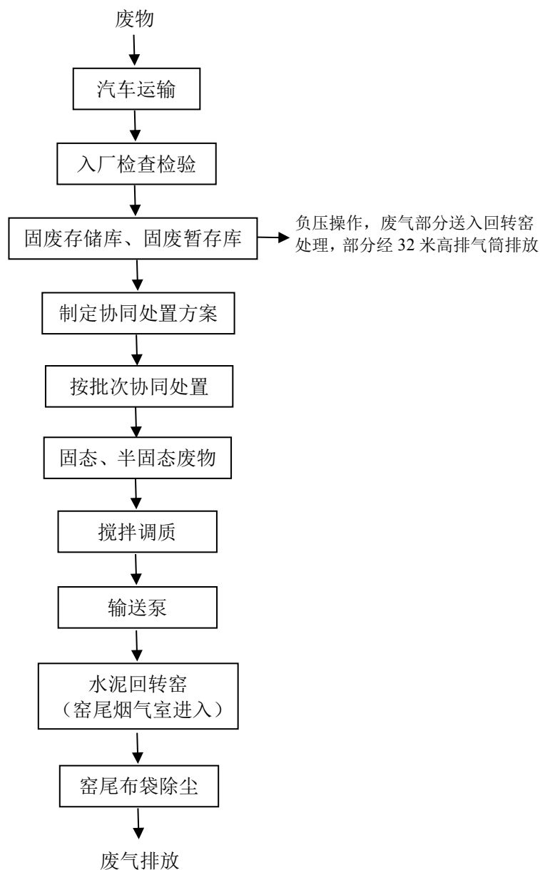
图 3-4 固体废物协同处置总体流程图
