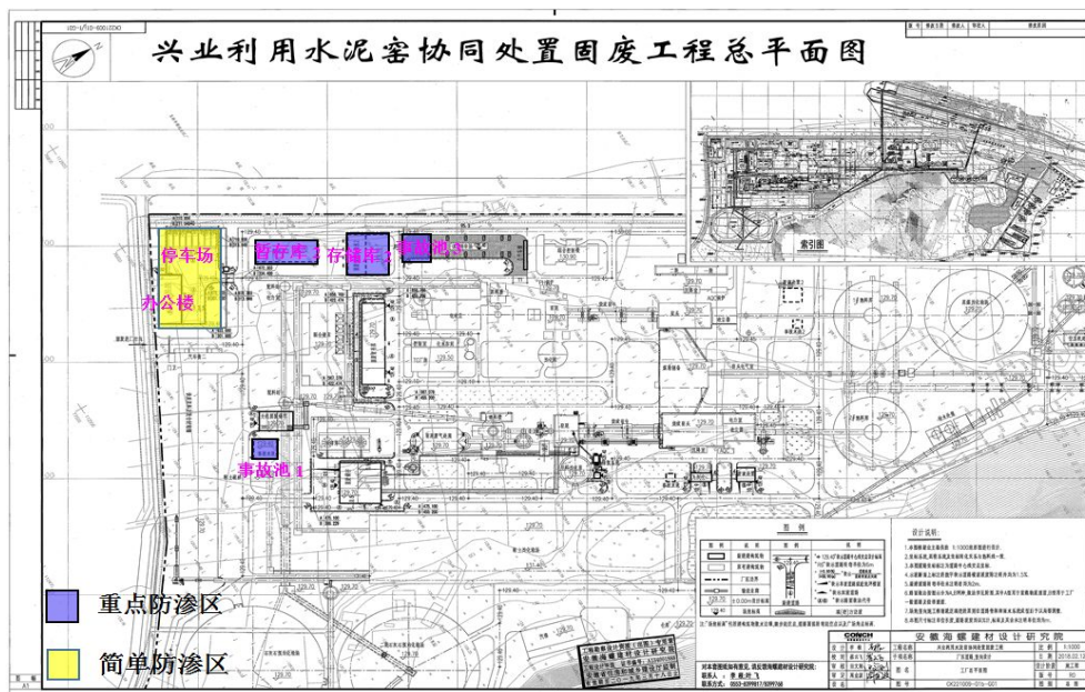
图 4-3 项目分区防渗图
