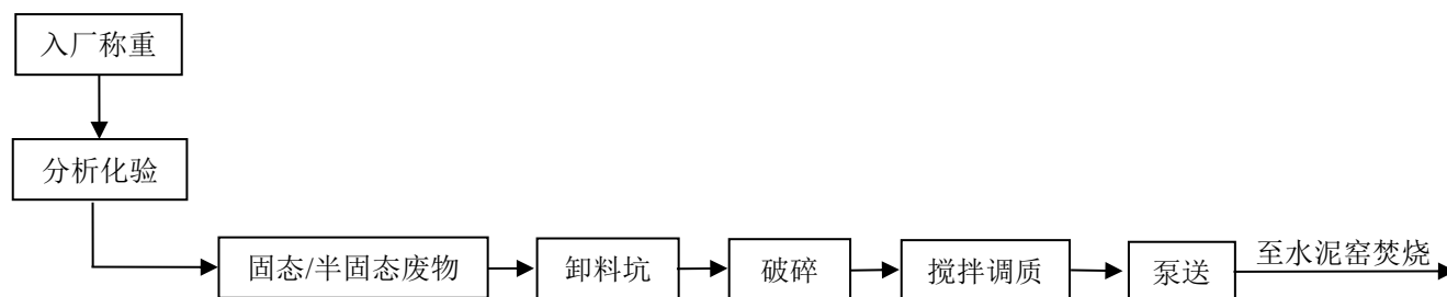
图 3-5 固态/半固态废物预处理流程
