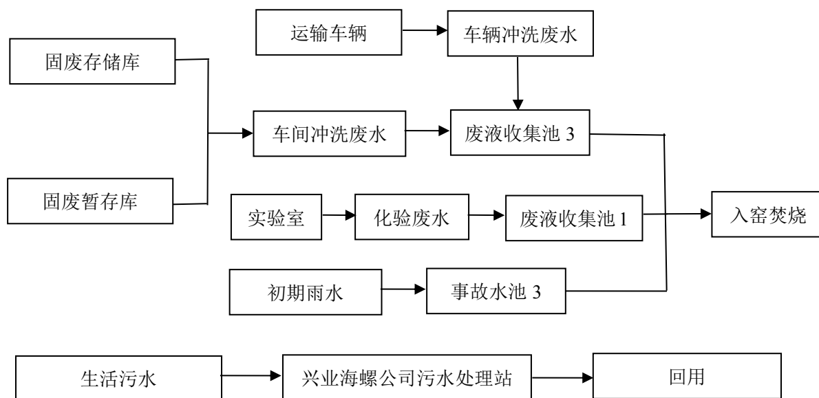
图 4-1 废水处理流程示意图
