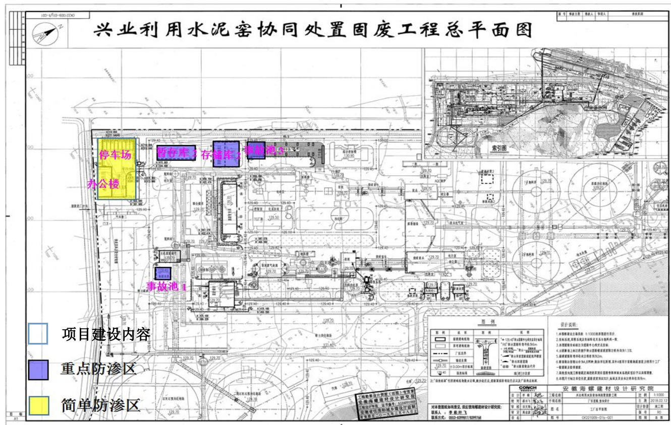
图 3-2 项目平面布置图
