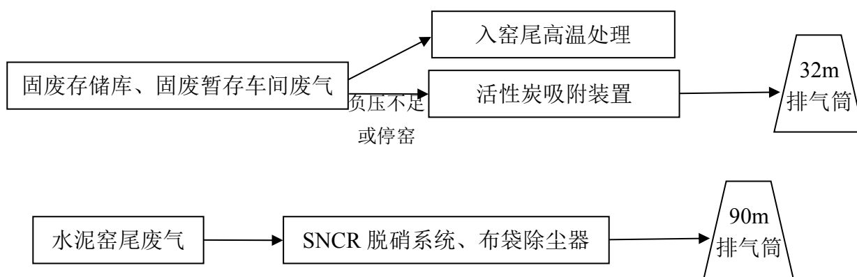
图 4-2 废气处理流程示意图
