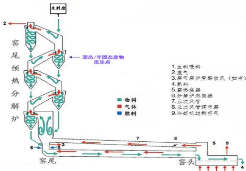
图 3-6 危险废物入窑位置示意图
