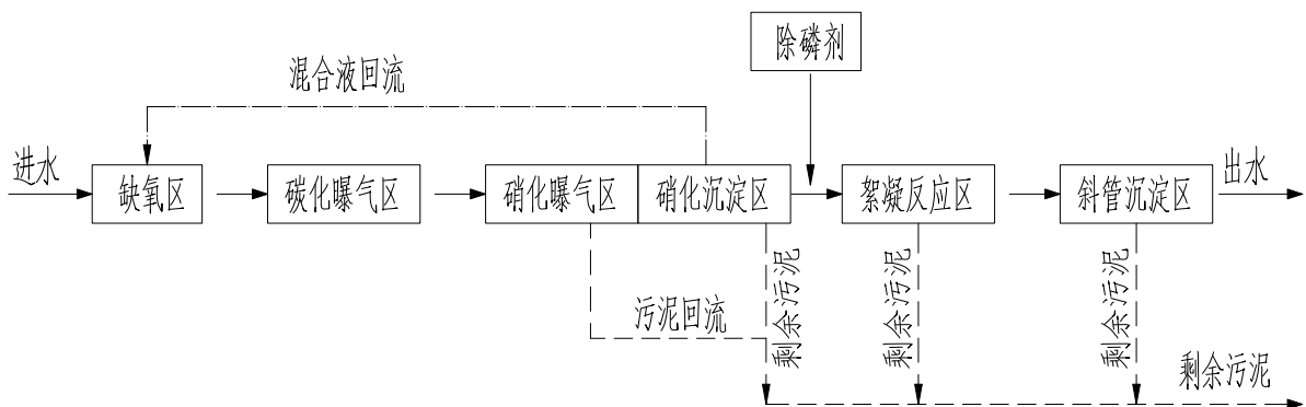
图 2-1 工艺流程及产污节点图
