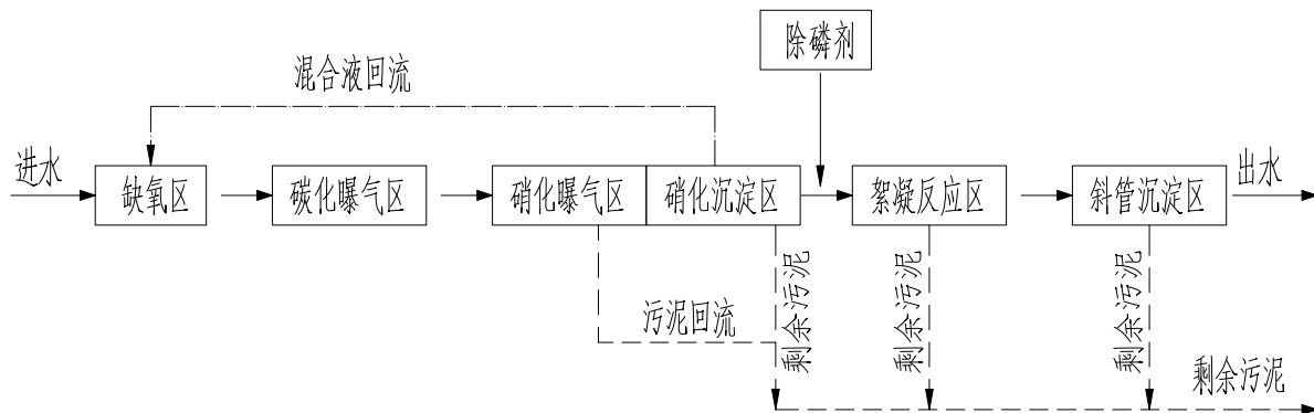
图 3-1 工艺流程及产污节点图
