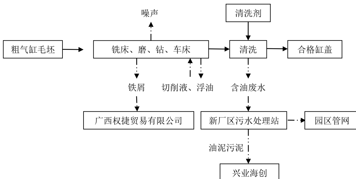
图4 工艺流程及产污环节图
