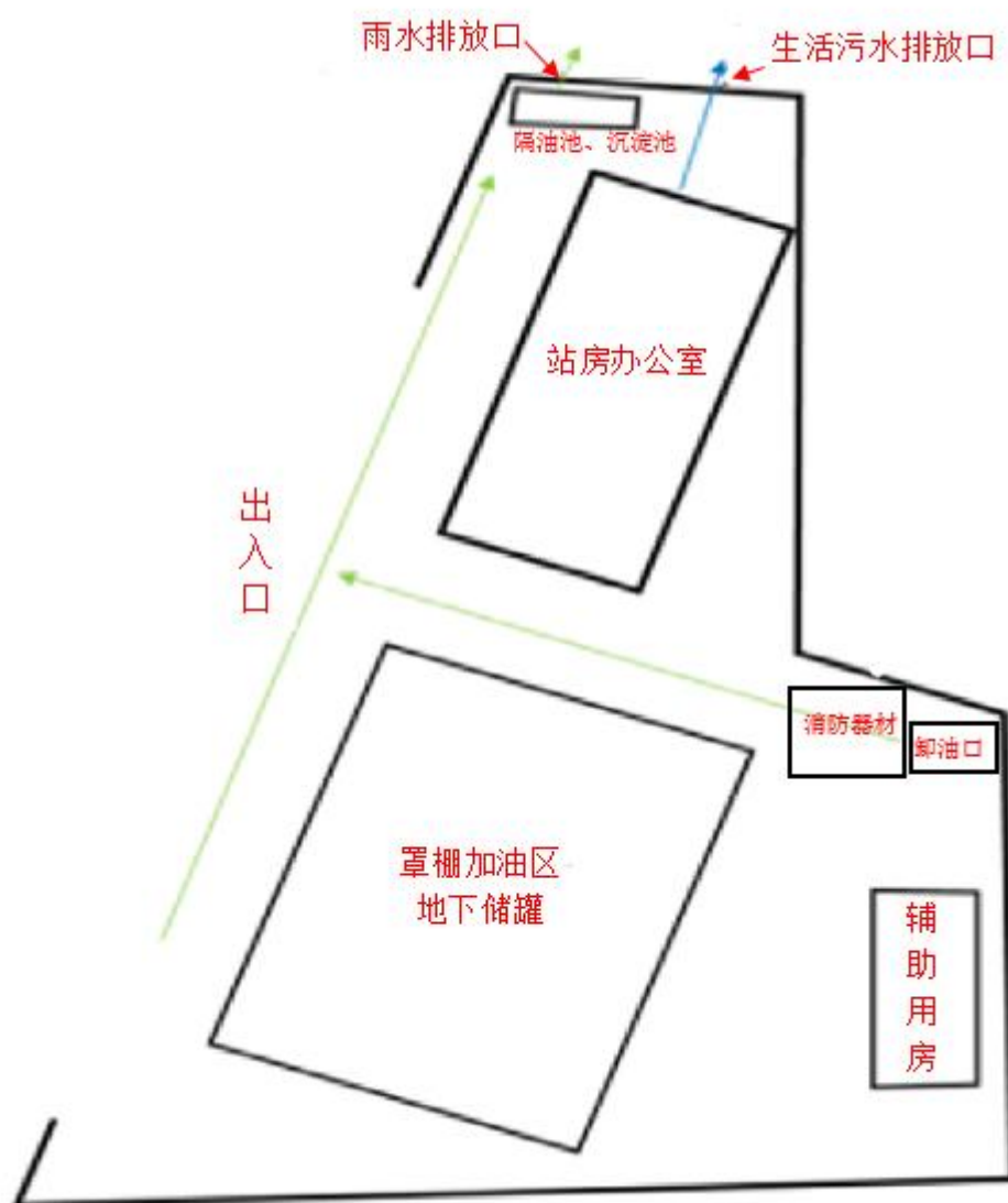
图 2-2 企业总平面布置图
