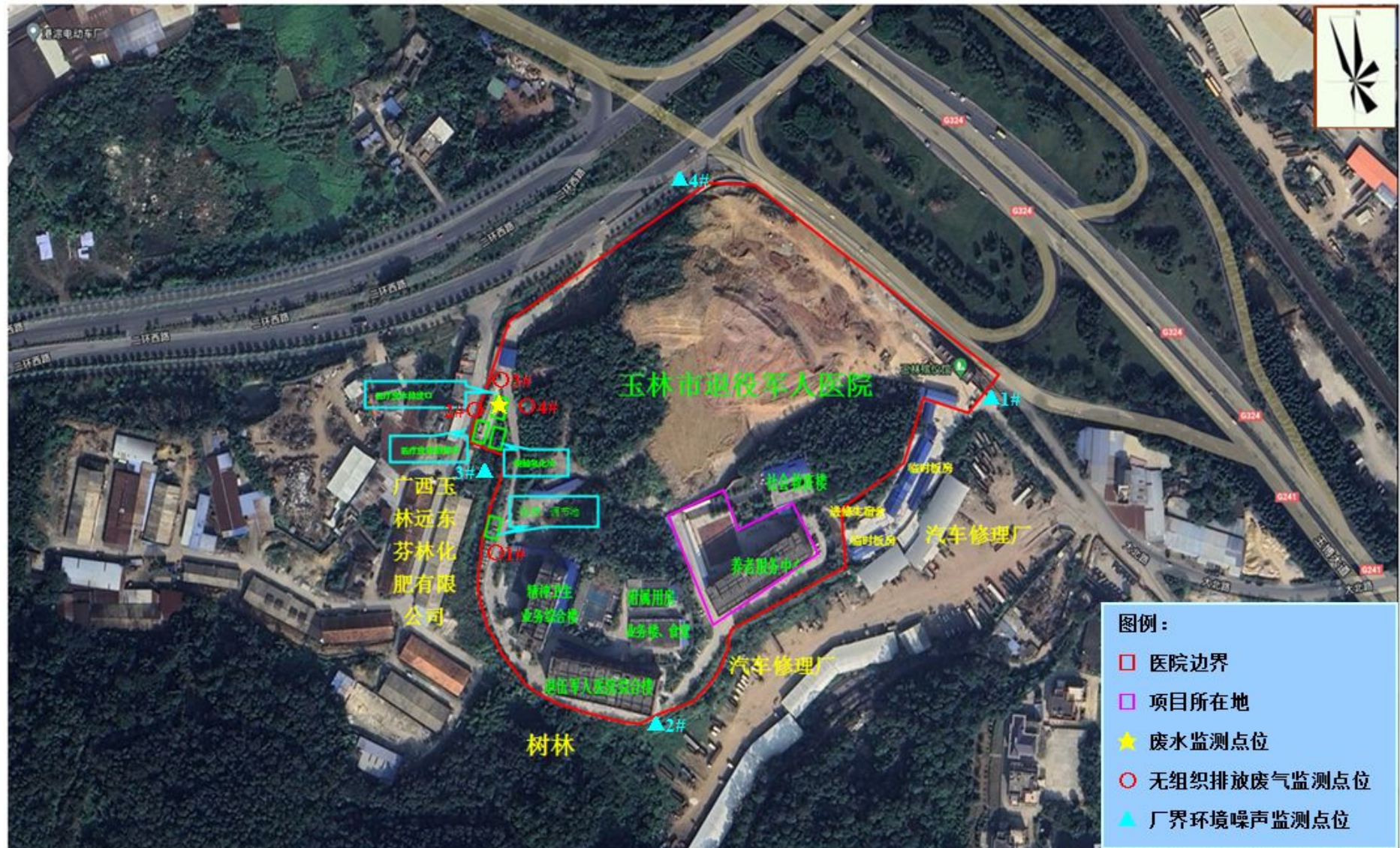
图 6-1 废水、废气、噪声监测点位图
